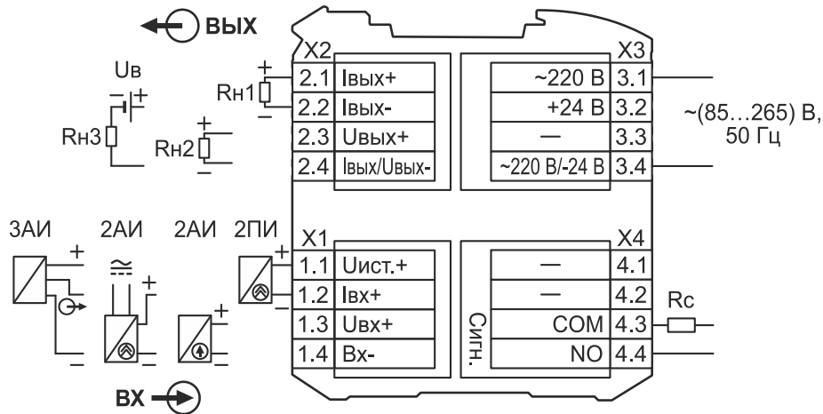
Рисунок 7 – Электрическая схема подключения преобразователей НПСИ-230-УНТ-Х-220-МХ
