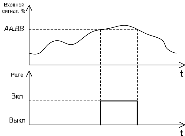
Рисунок 2 – Прямая функция. Реле срабатывает, если входной сигнал больше уровня сигнализации, сброс реле, если меньше
