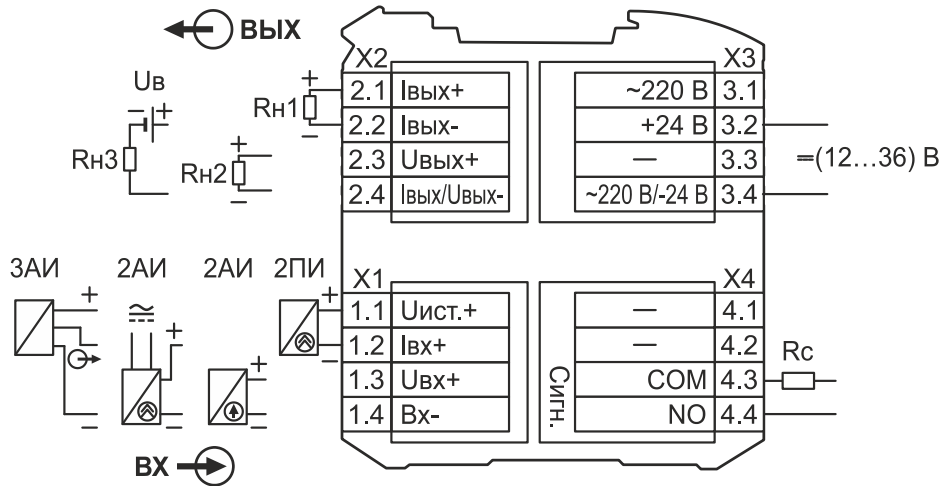
Рисунок 8 – Электрическая схема подключения преобразователей НПСИ-230-УНТ-X-24-MX
